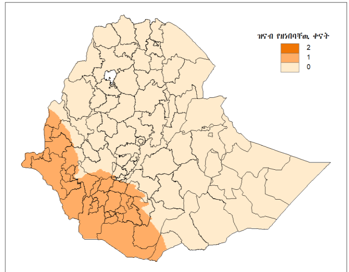
ካርታ 2 እ.ኤ.አ ከዲሴምበር 11 እስከ 20/2024 ድረስ ዝናብ የዘነበባቸው ቀናት
