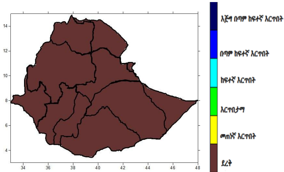
ካርታ 5 እ.ኤ.አ ከዲሴምበር 1 እስከ 10/2024 ድረስ የነበረው የእርጥበት ሁኔታ
