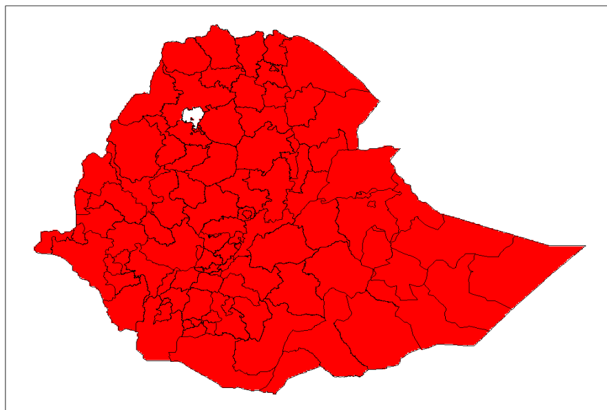
የዝናብ የዝናብ መጠን ከረጅም ጊዜ አማካይ ጋር ሲነፃፀር ከመደበኛ በታች መደበኛ ከመደበኛ በላይ
