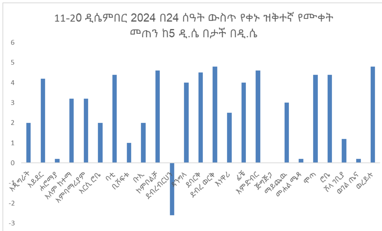
ምስል 1፡ የቀኑ ዝቅተኛ የሙቀት መጠን በዲ.ሴ
