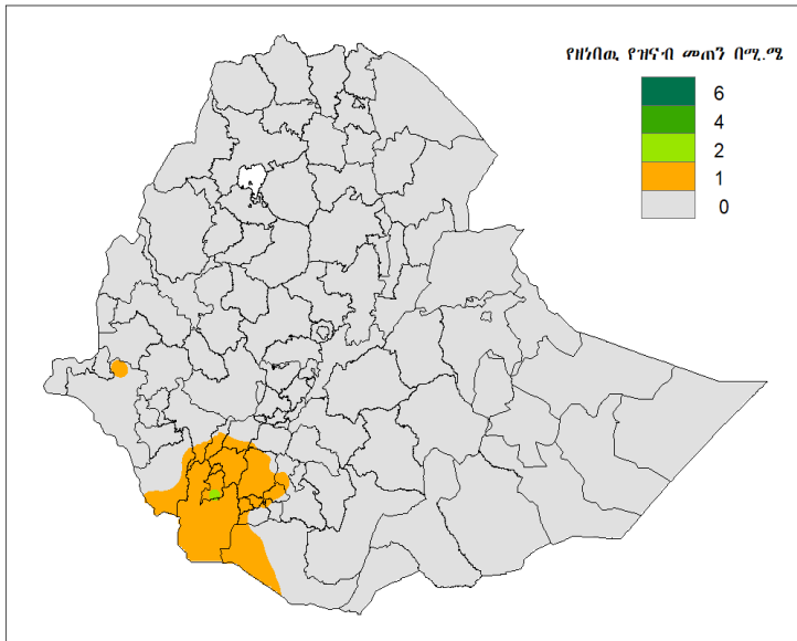
ካርታ 1 እ.ኤ.አ ከዲሴምበር 11 እስከ 20/2024 ድረስ የነበረው የዝናብ መጠን በሚ.ሜ
