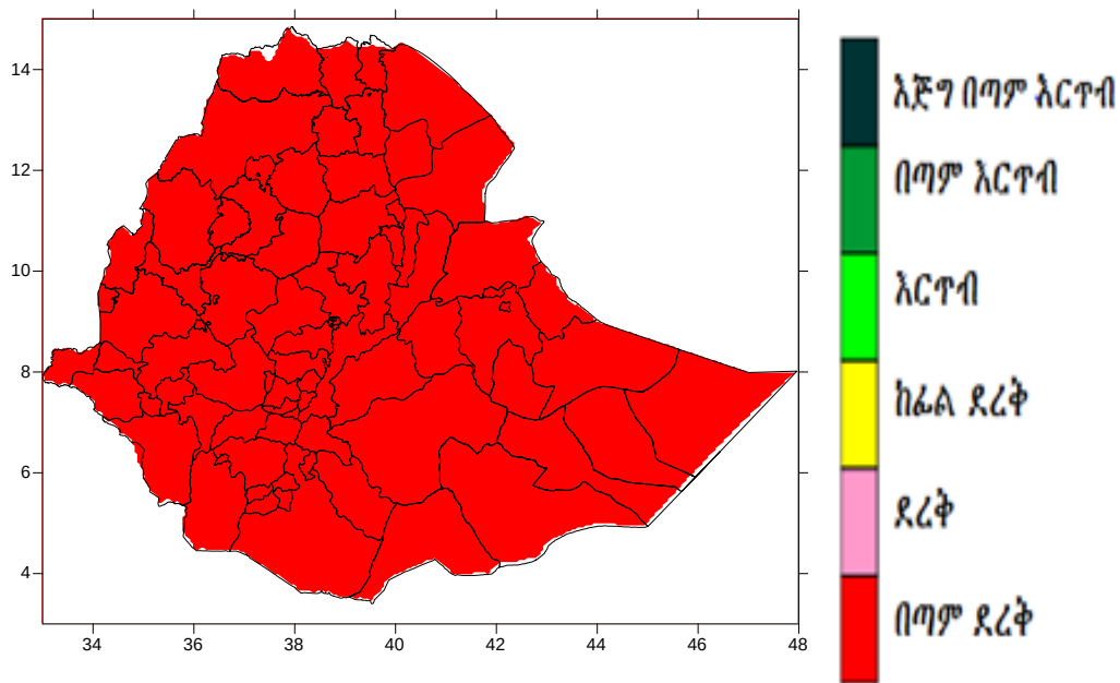
ካርታ 4 እ.ኤ.አ ከዲሴምበር 11 እስከ 20/2024 ድረስ የነበረው የእርጥበት ሁኔታ
