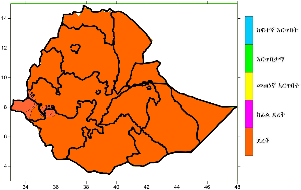
ካርታ 5. እ.ኤ.አ ከዲሴምበር 11-20/2017 በተፋሰሶች ላይ የነበረው የእርጥበት መጠን
